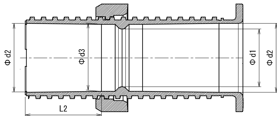
断面 A-A
